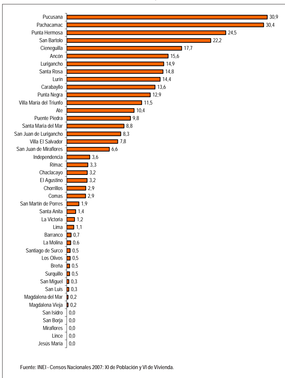
GRÁFICO N° 4.16 PROVINCIA DE LIMA: VIVIENDAS PARTICULARES CON OCUPANTES PRESENTES QUE NO TIENEN DISPONIBILIDAD DE ALUMBRADO ELÉCTRICO POR RED PÚBLICA, SEGÚN DISTRITO, 2007 (Porcentaje)
