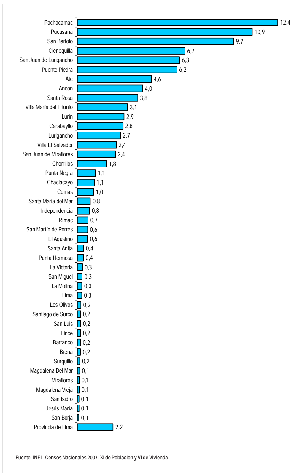
GRÁFICO N° 4.4 PROVINCIA DE LIMA: VIVIENDAS PARTICULARES QUE SON VIVIENDA IMPROVISADA CON PERSONAS PRESENTES, SEGÚN DISTRITO, 2007 (Porcentaje)
