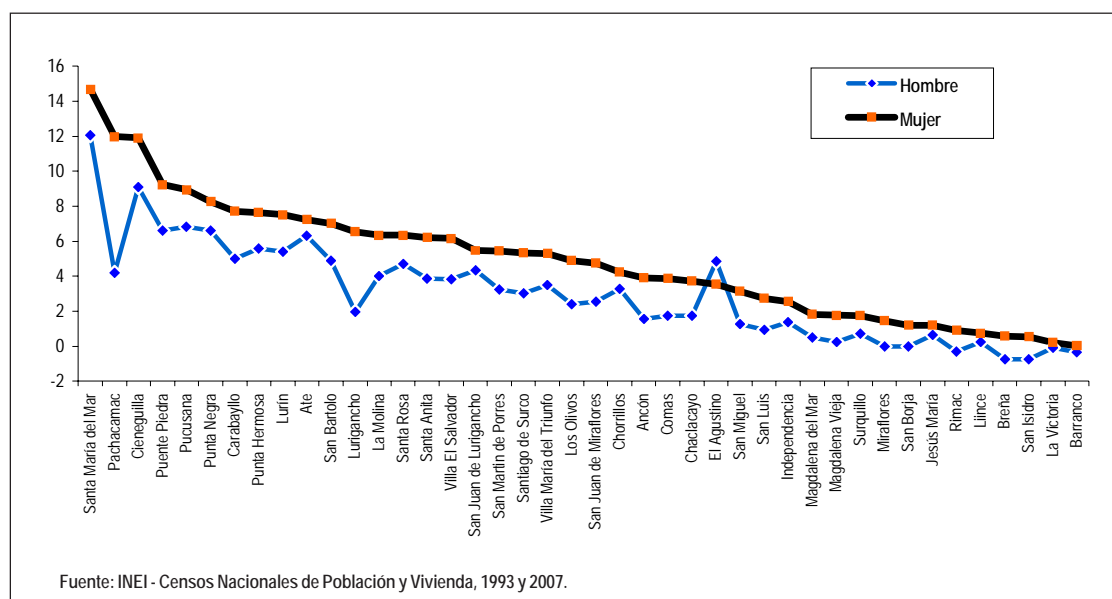
GRÁFICO N° 3.2 PROVINCIA DE LIMA: TASA DE CRECIMIENTO PROMEDIO ANUAL DE LA PEA FEMENINA Y MASCULINA, SEGÚN DISTRITO Y PERÍODO INTERCENSAL, 1993 Y 2007 (Porcentaje)
